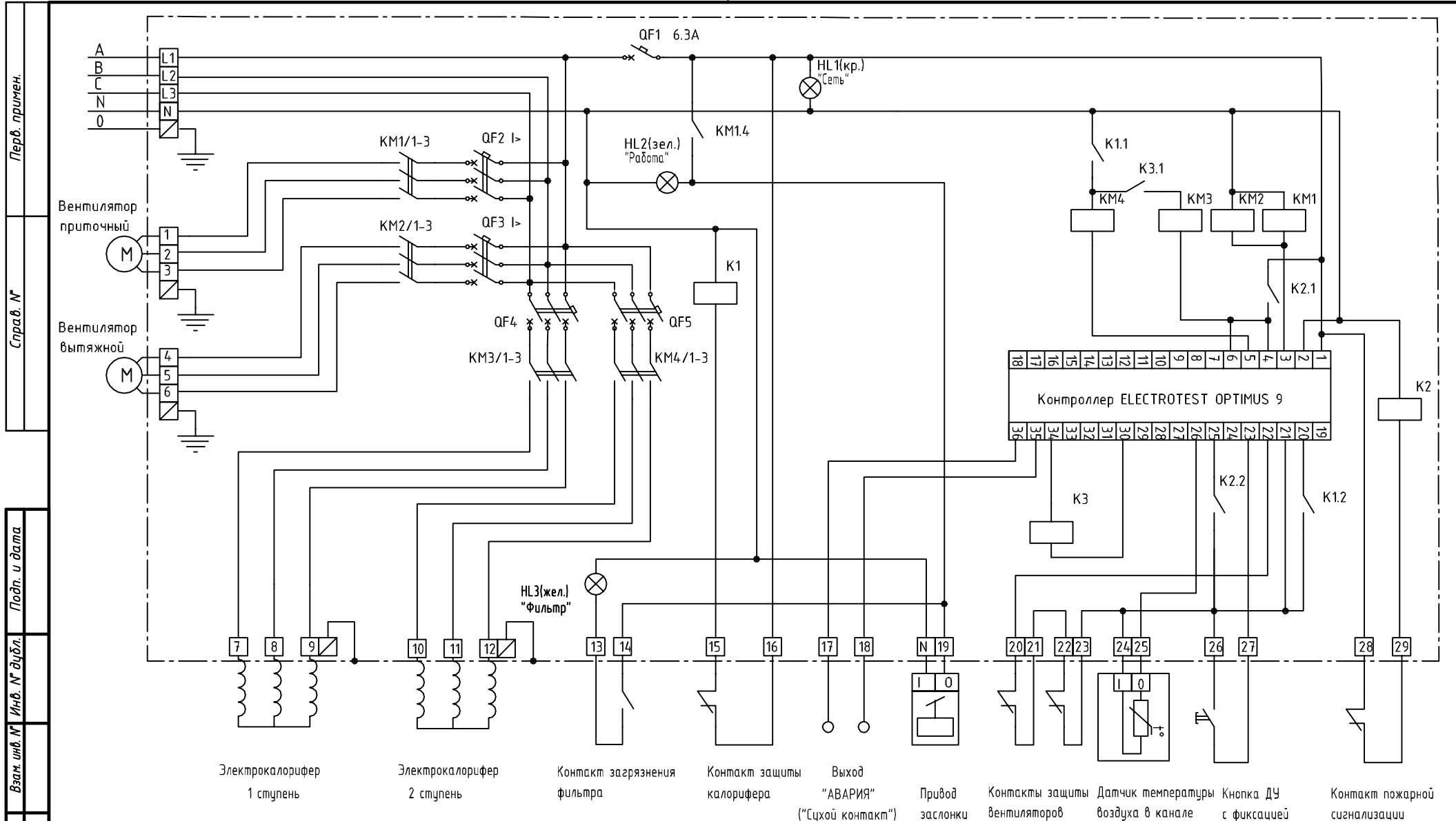
Схема электрическая принципиальная Optimus9 / Электро 4
