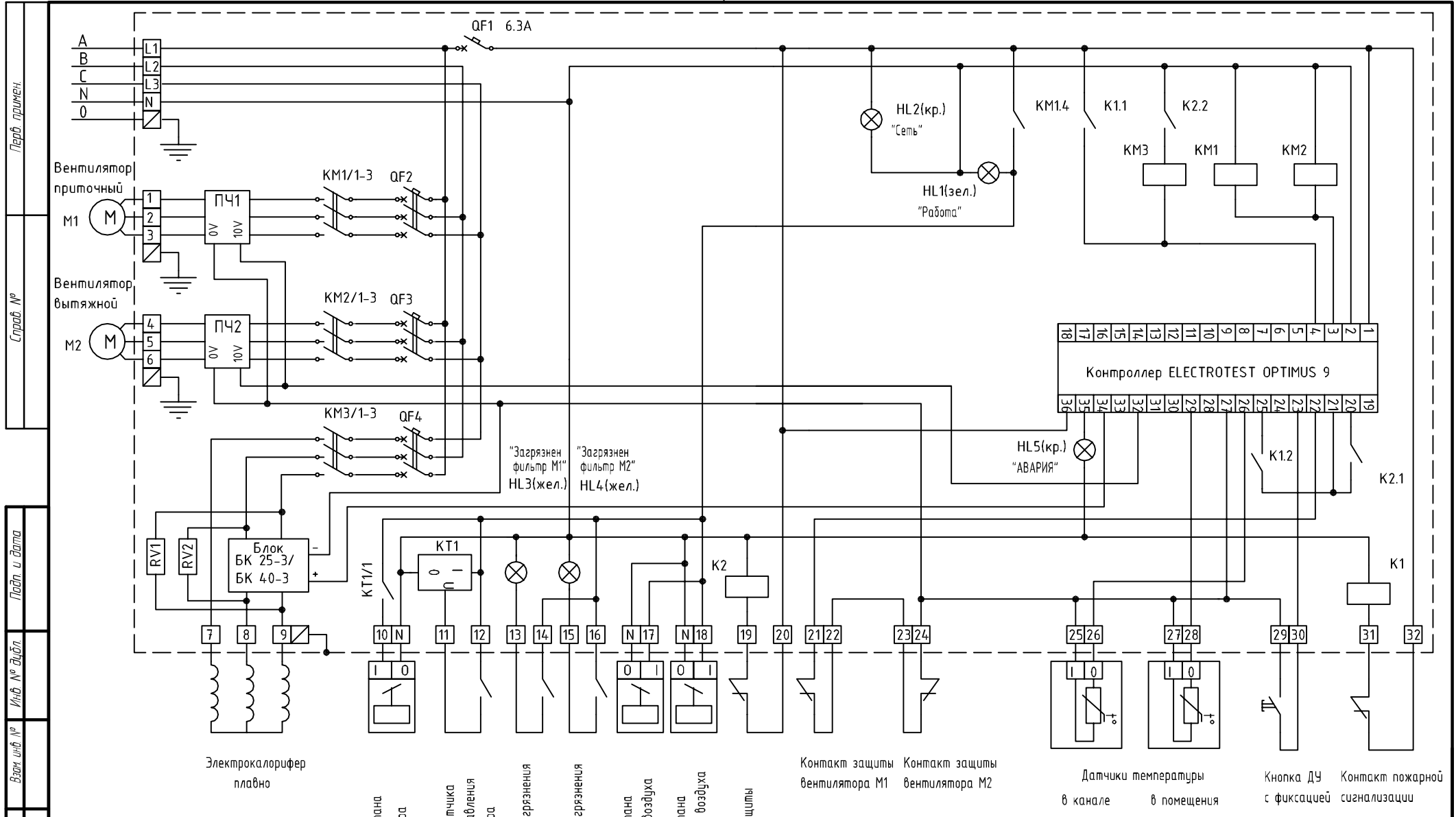
Схема электрическая принципиальная Optimus9 / Комби 5
