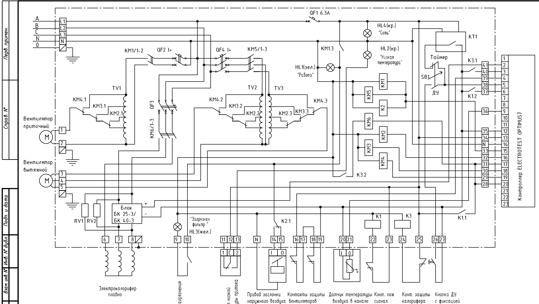
Схема электрическая принципиальная Optimus7 / Электро 7
